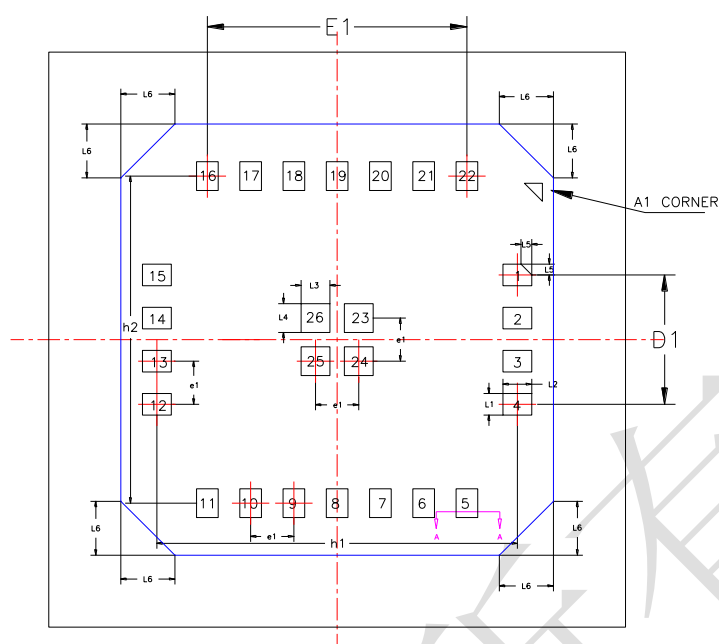
图 5-3 Bottom View
