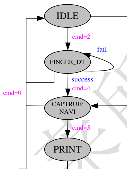
图 4-9 芯片状态图
