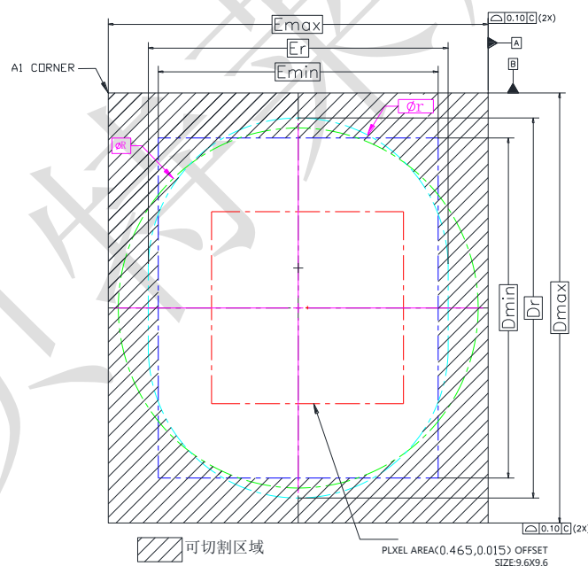
图 5-7 Top View
