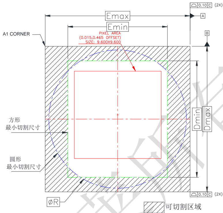
图 5-10 Top View
