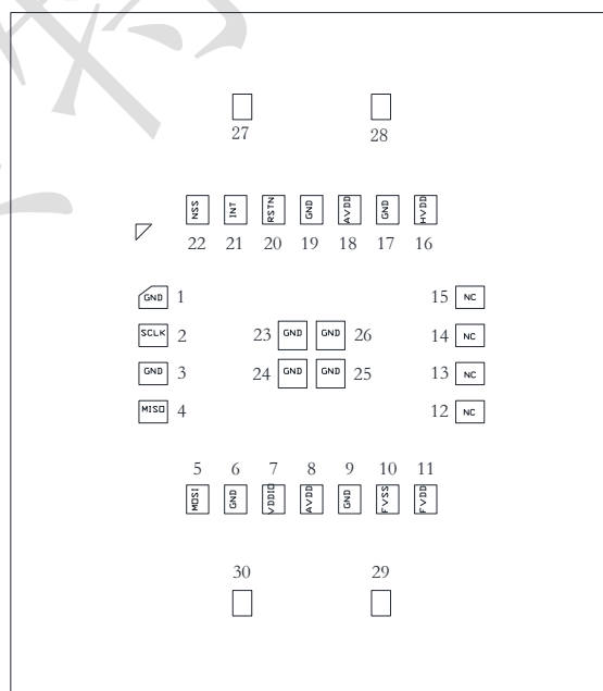
图 1-2. BF81192C_X 管脚排列示意图(Top View)
