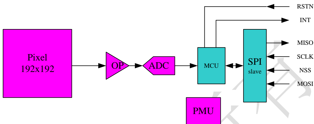
图 3-1 原理方框图
