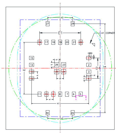
图 5-9 Bottom View
