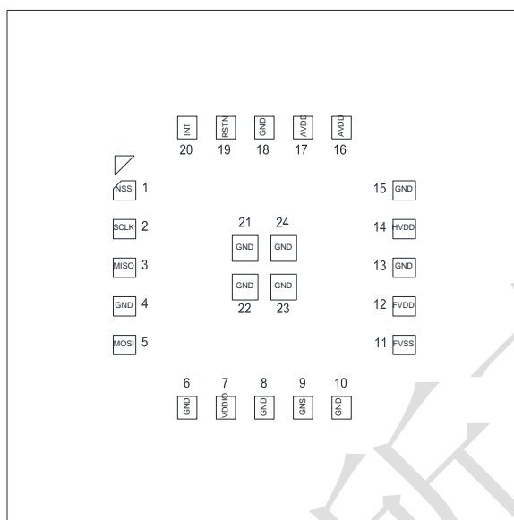
图 1-3. BF81192D_X 管脚排列示意图 (Top View)
