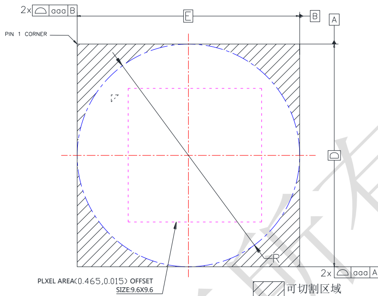
图 5-4 Top View
