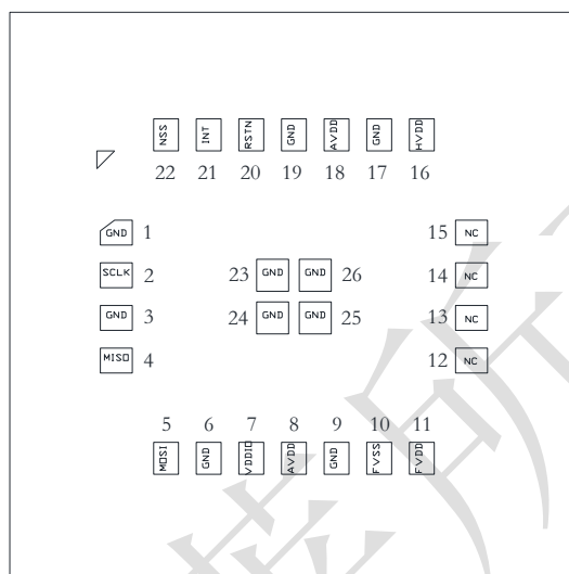
图 1-1. BF81192A_X, BF81192B_X 管脚排列示意图(Top View)
