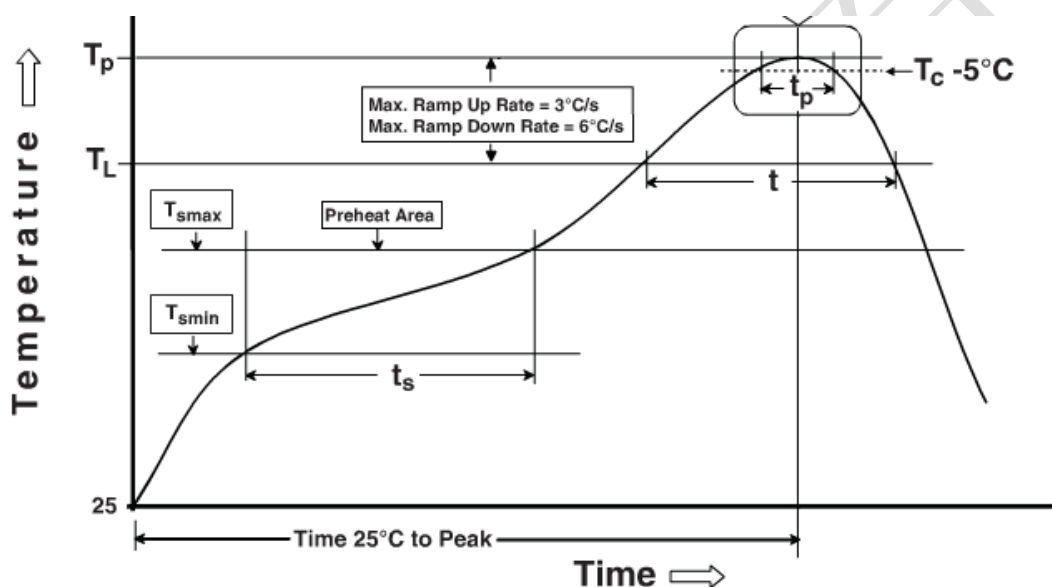
图 2-1. BF81192X_X ReflowTp. 曲线图
