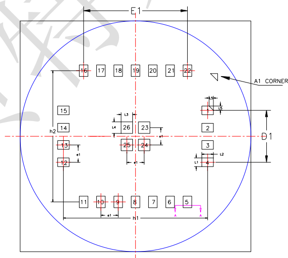
图 5-6 Bottom View
