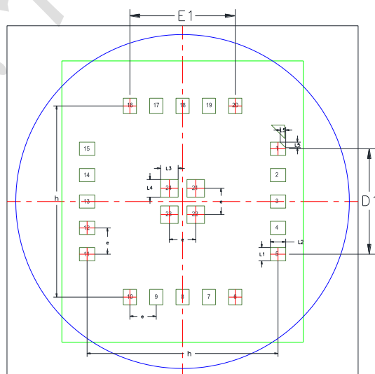
图 5-9 Bottom View
